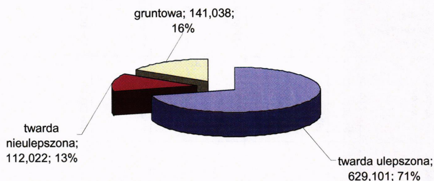
Wykres 5. Nawierzchnie dróg powiatowych (km/%)
